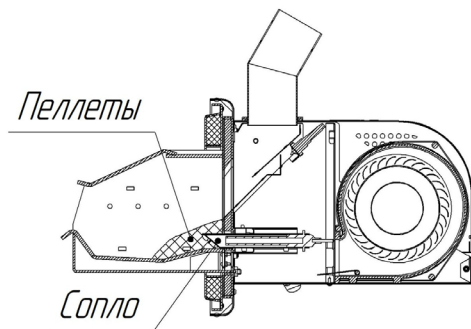
Рисунок 11 – Ручная загрузка топлива для розжига
