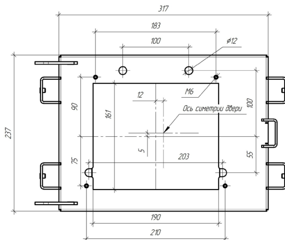
Рисунок 20 - Разметка проема и мест крепления ГПФ-42 (3.0)
