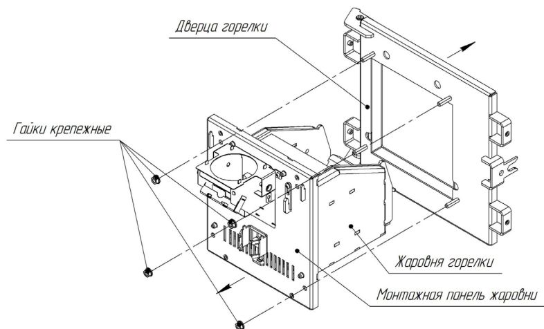
Рисунок 18 - Демонтаж двери
